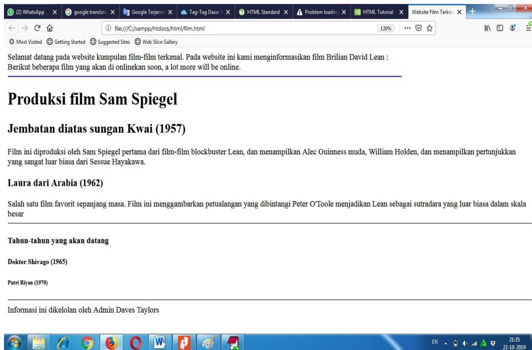
Gambar 4 Tampilan Latihan 1
