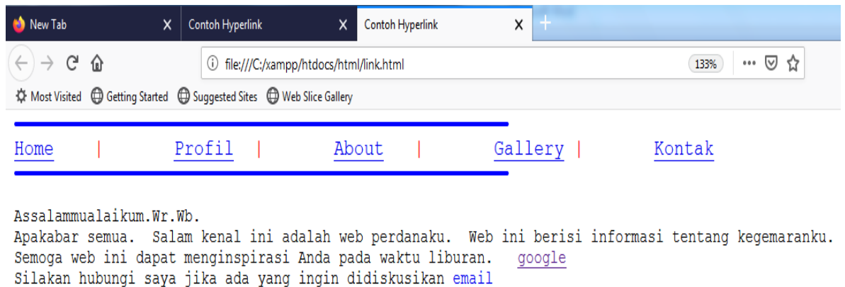
Gambar 17 Tampilan Hyperlink
