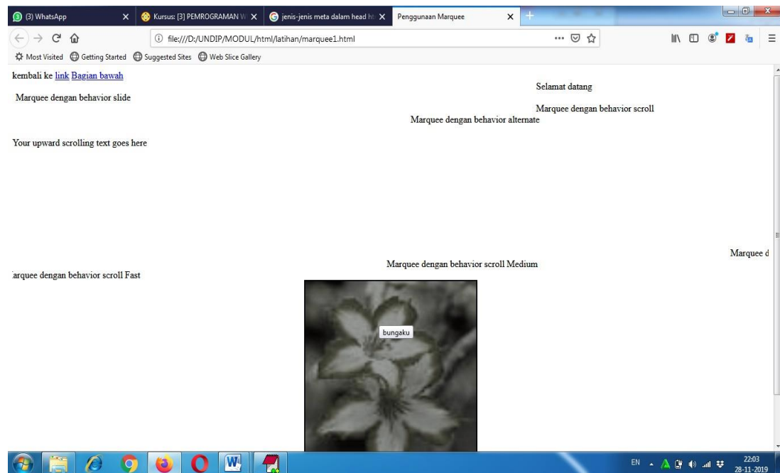
Gambar 8 Tampilan Marquee
