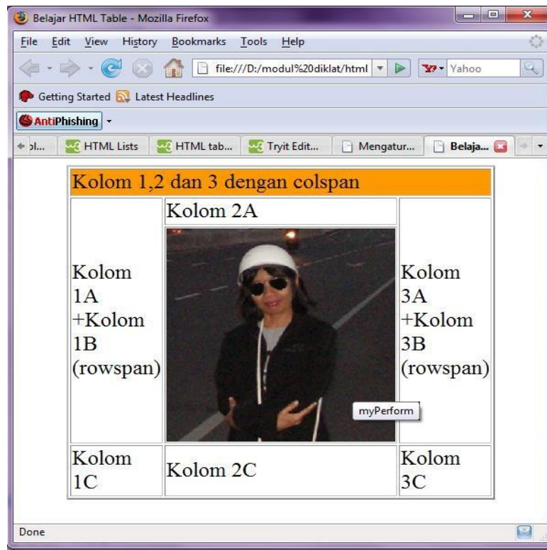
Gambar 21 Latihan Tabel
