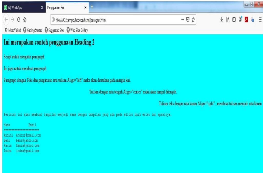
Gambar 5 Tampilan Latihan 4
