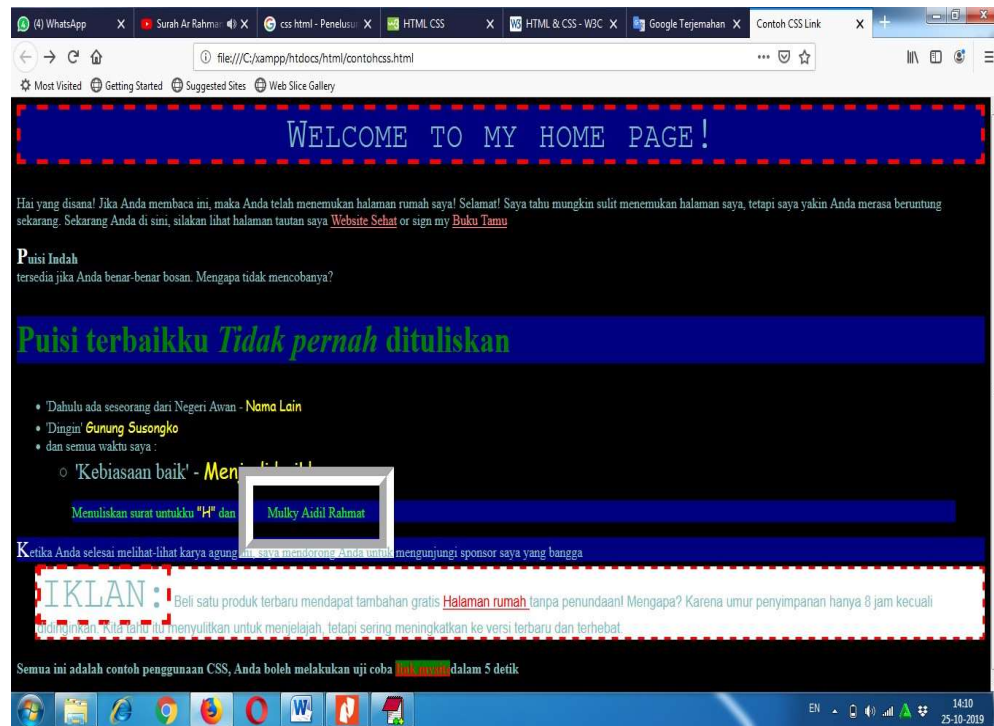
Gambar 32 Latihan CSS
