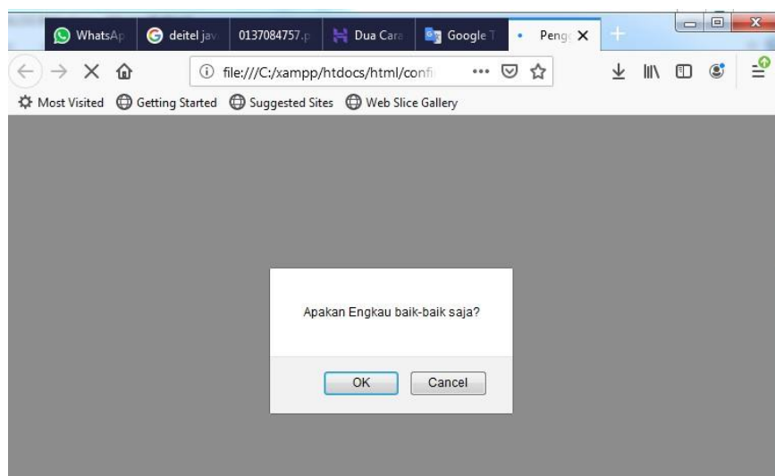
Gambar 44 Tampilan konfirmasi
